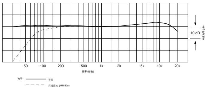
频率特性
