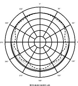
指向特性
