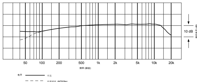
频率特性
