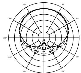
声压曲线1制度5 dB
