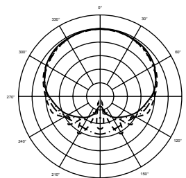
指向特性
