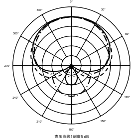
指向特性
